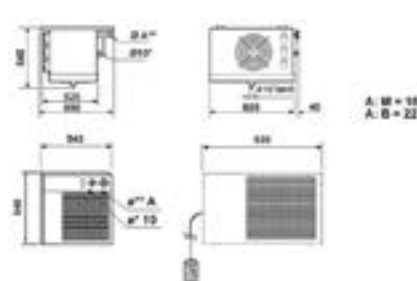
Wymiary dla serii MDB4... BDB4
