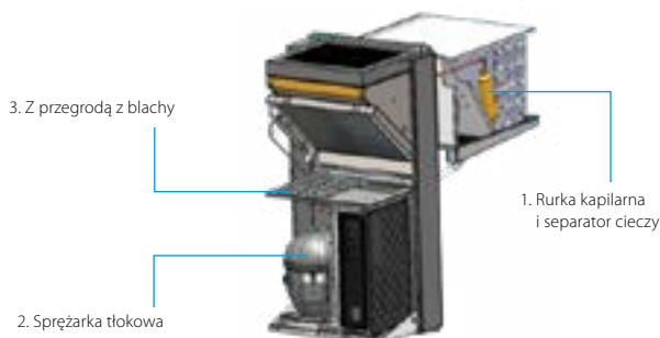
GM z tradycyjnymi czynnikami chłodniczymi
