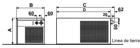
Agregat zewnętrzny dla serii RDV2
