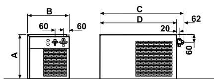
Agregat zewnętrzny dla serii RDV1
